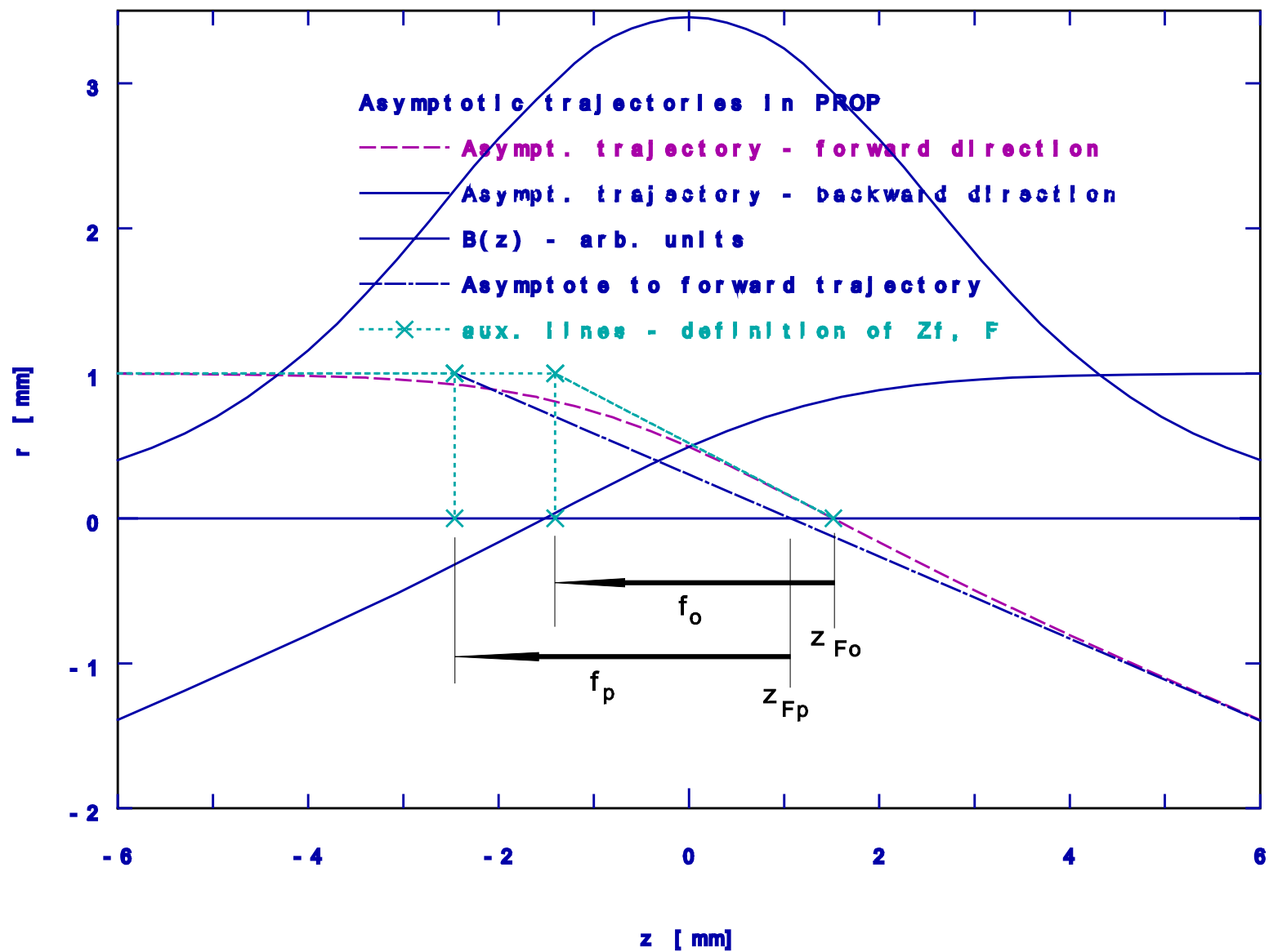
Definice optických vlastností objektivu a projektivu (případ magnetické čočky).
